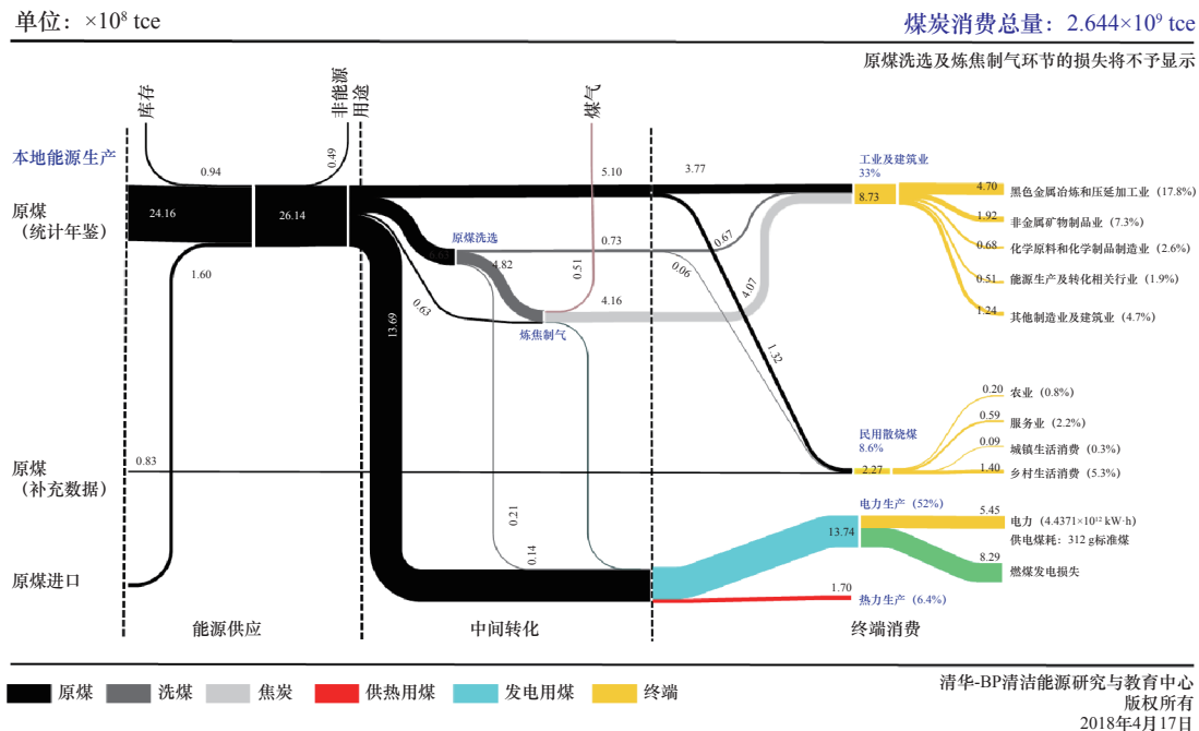
图 1 2016 年我国煤炭直接消费流向图
